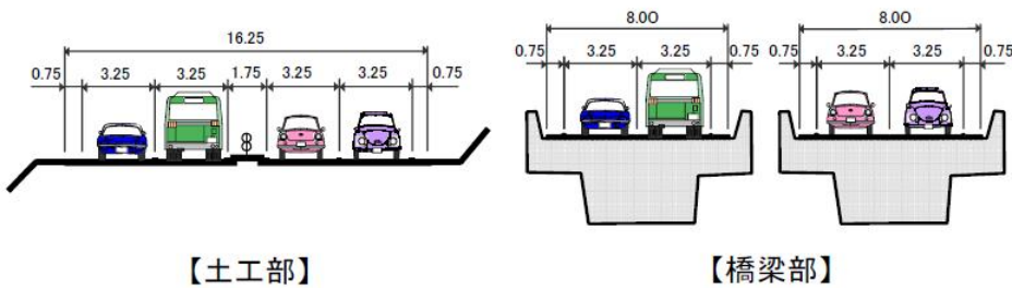
▲標準断面図 (単位:m)
