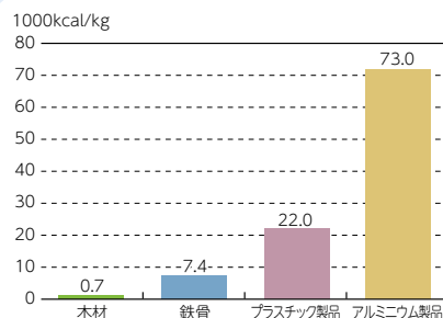
住宅用資材の製造に必要なエネルギー (推計) 資料：科学技術庁「ライフサイクルエネルギーに関する調査研究」
