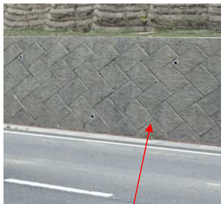
視覚的影響低減のための 粗面コンクリートブロック積工
