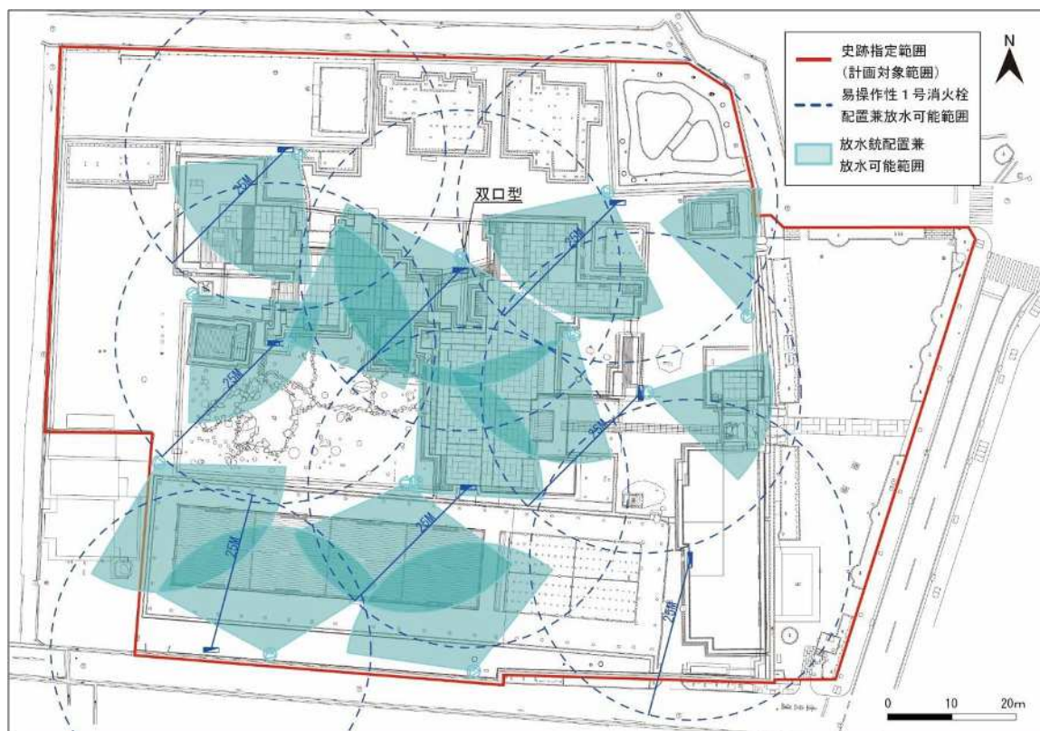
図 9 - 2 消火設備設置位置
