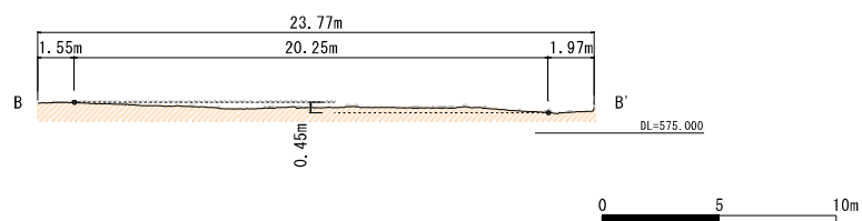
図 8－3 池泉庭園の断面図
