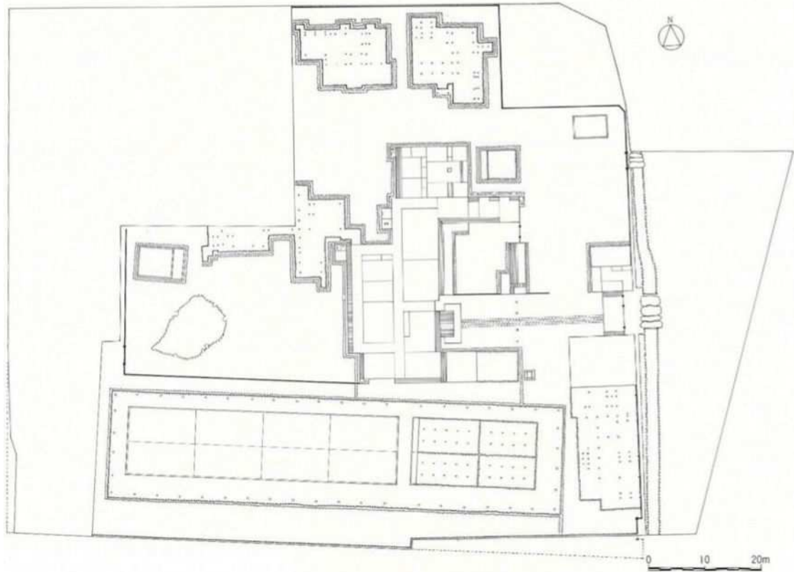
図 3－9 第一次・第二次整備竣工平面図
