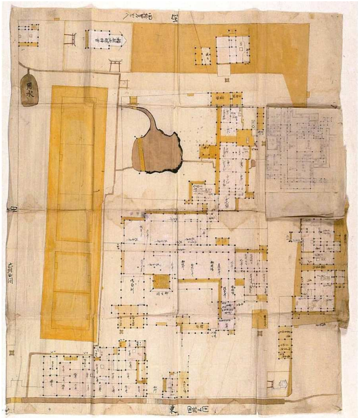
写真 3-3 文政 13 年 御勝手方御建替御普請皆出来形掛絵図面
