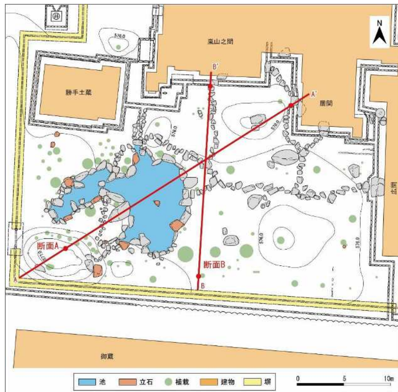
図 8－2 池泉庭園平面図
