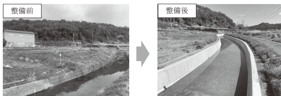
農業用水路（肥田瀬用水）の予防保全対策（関市）
