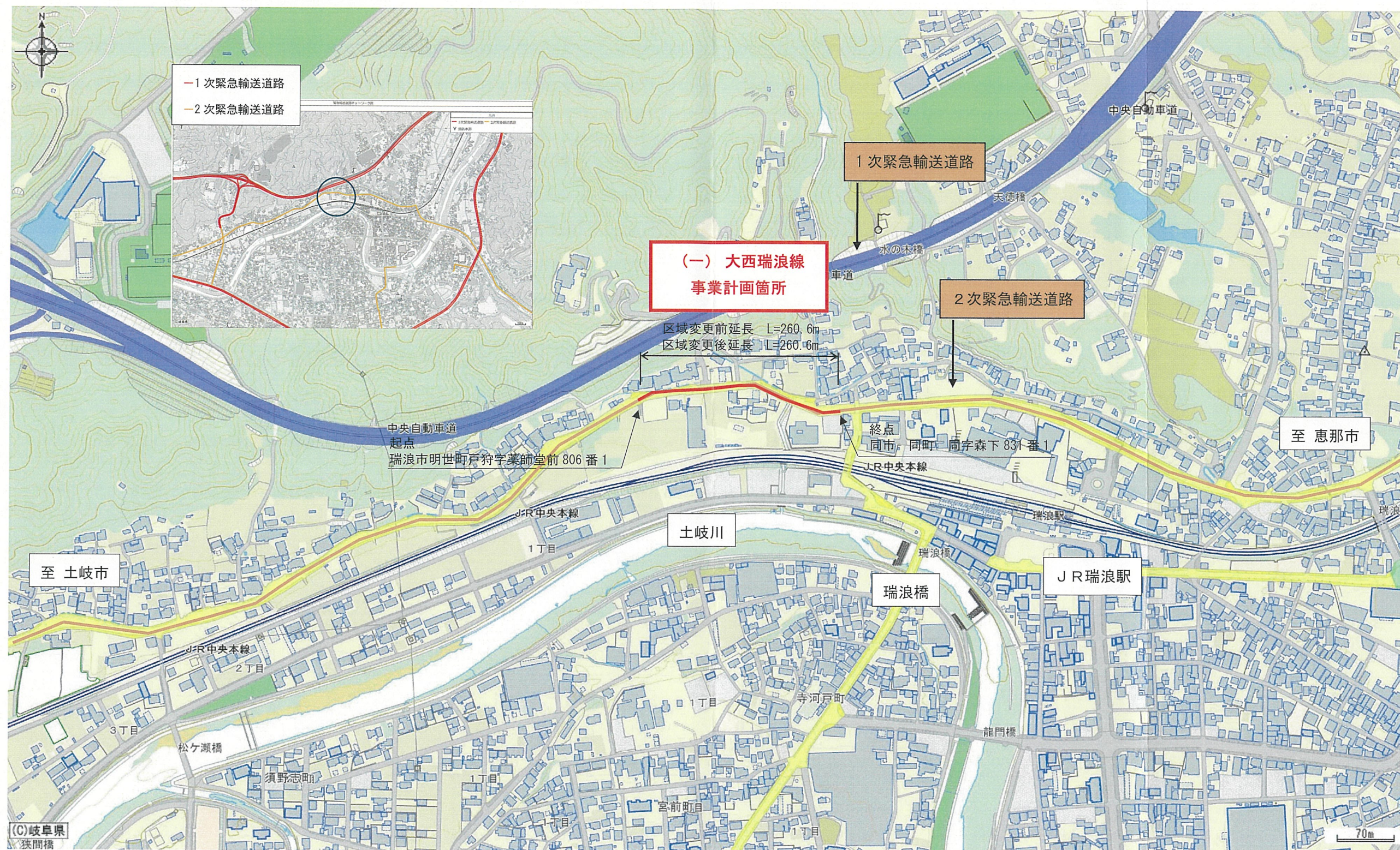
詳細位置図 S=1/5,000
