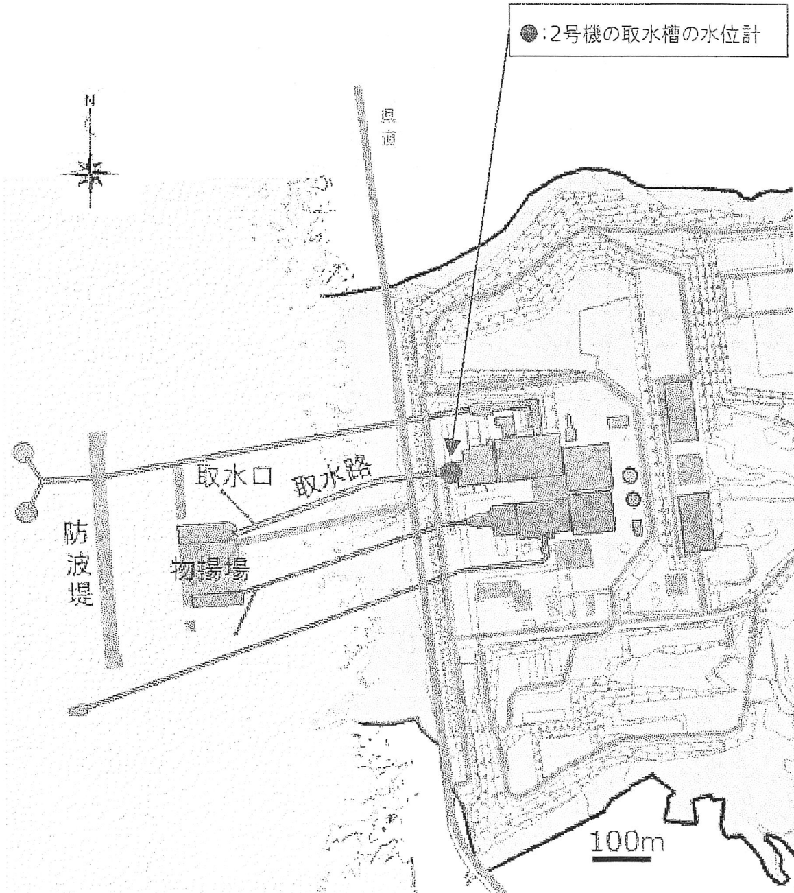
志賀原子力発電所 構内図
