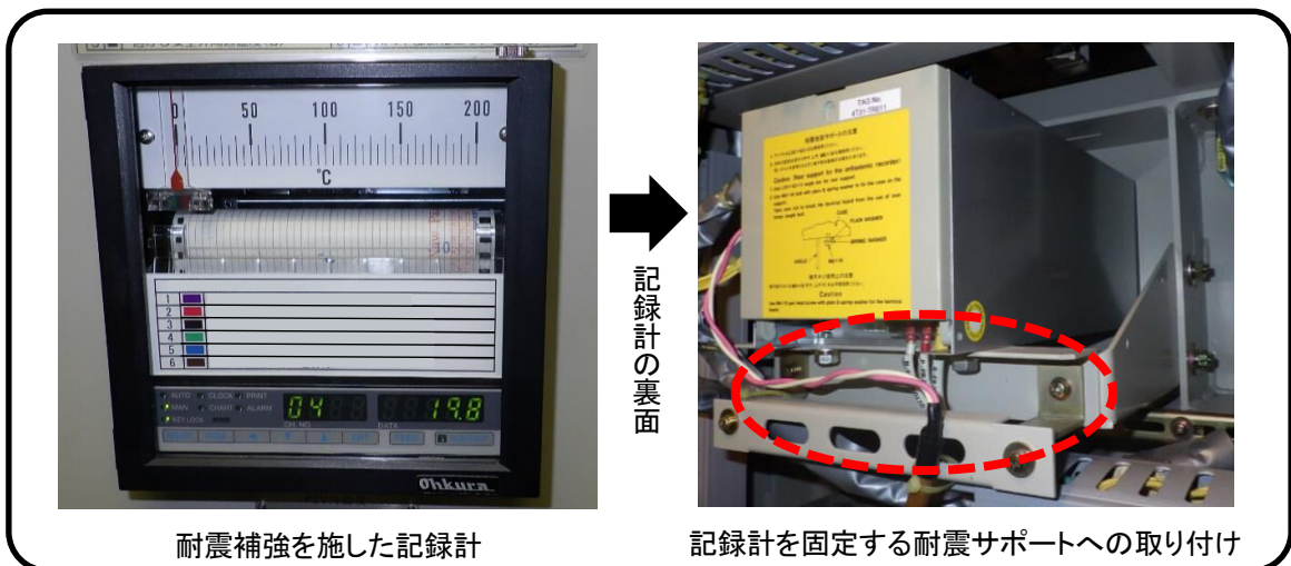
耐震補強対策の一例
