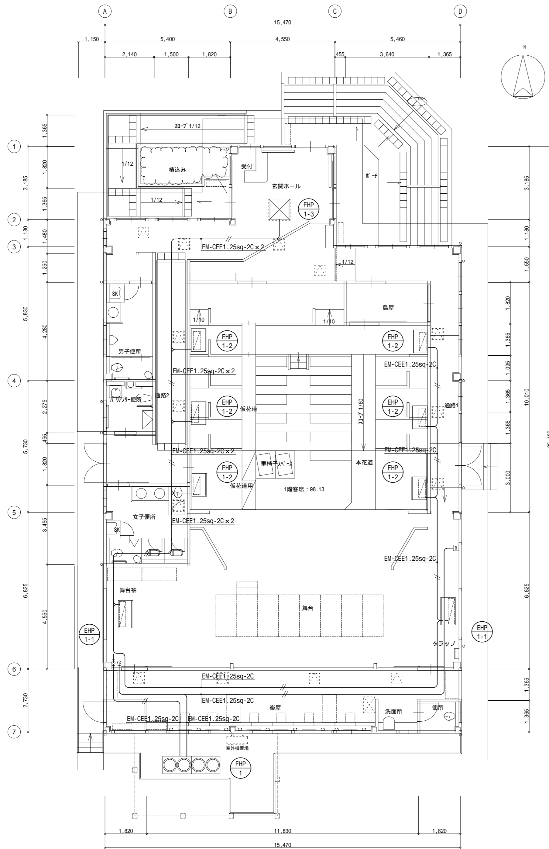
改修後空調設備平面図 S=1/100
