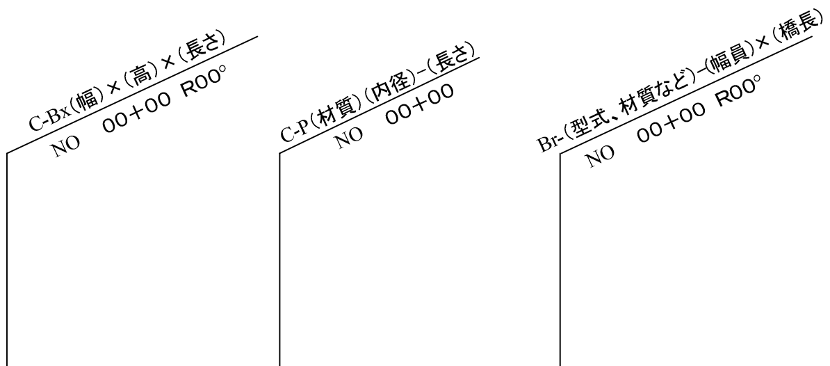
解説 図 2-3 横断構造物の旗上げ表現(例)
