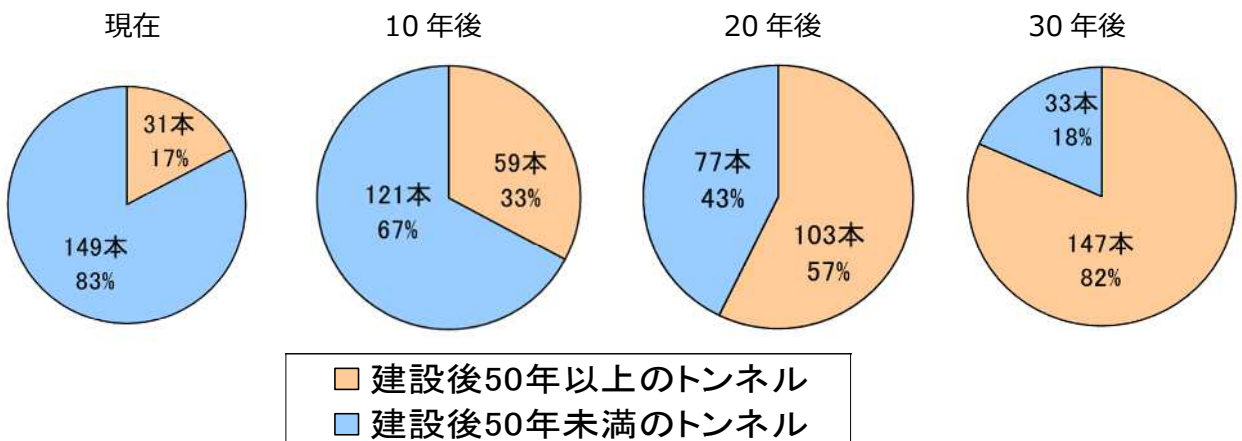
図 - 2. 建設後 50 年以上のトンネル本数の推移 (2024 年時点)
