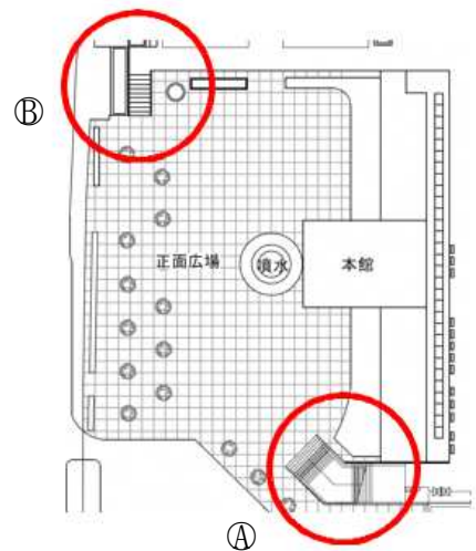
メモリアルセンター正面広場平面図
