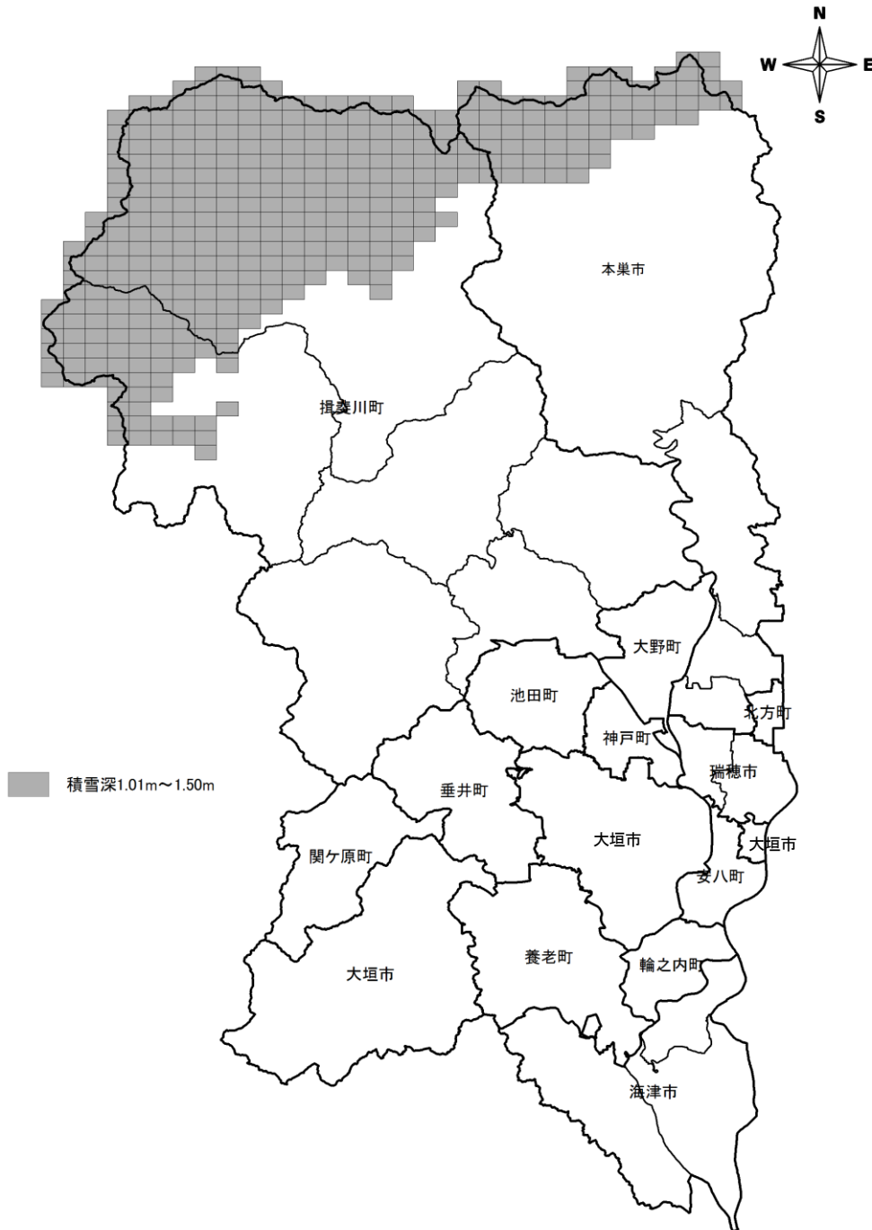
図2-1-1 最深積雪深図
