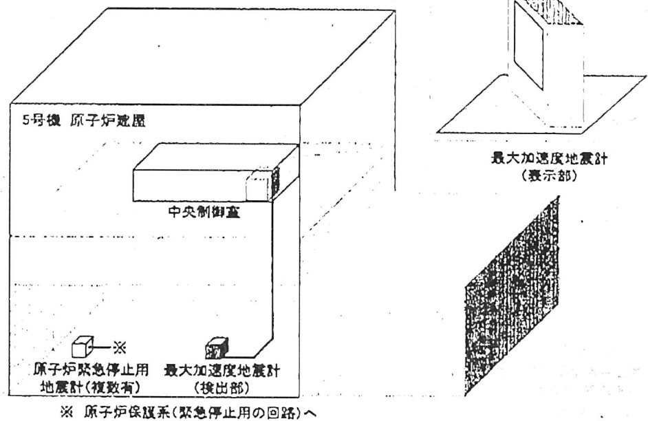
最大加速度地震計の概略図
