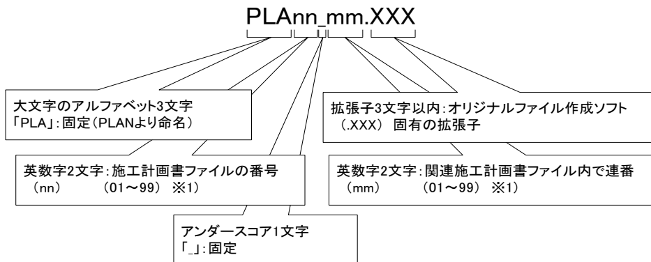
図 6-2 施工計画書オリジナルファイルの命名規則
