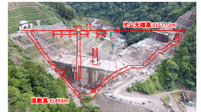
④ ダムサイト状況(上流上空より望む)
