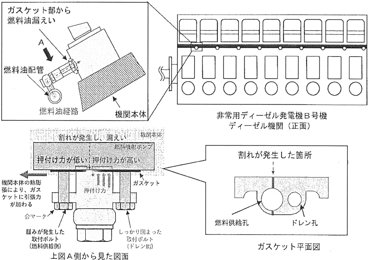
非常用ディーゼル発電機 燃料油配管概略図
