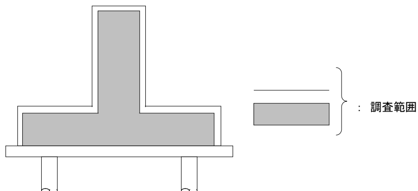
図-3 橋梁下部
