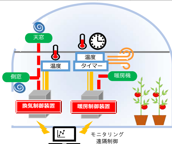
機器単独環境制御イメージ図
