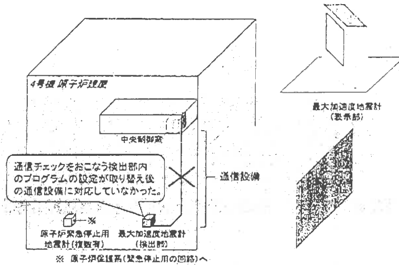
事象の概要図(4号機最大加速度地震計の例)
