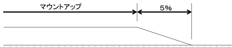
図1-6 マウントアップ歩道の摺付
