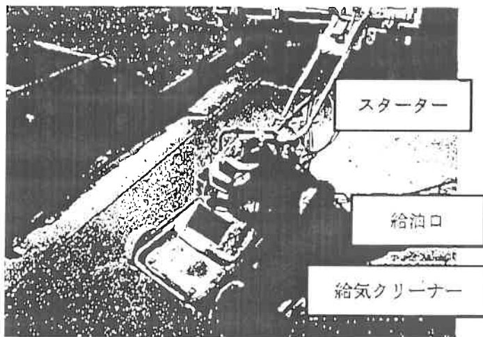
出火後の状況 (草刈機)
