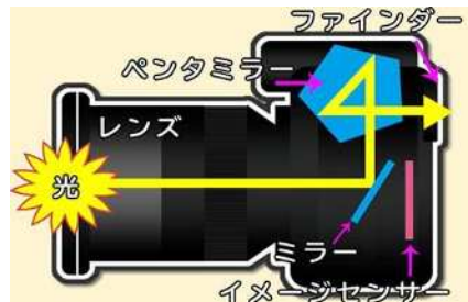
付録1-図1.1デジタル一眼レフカメラの構造 ※6
