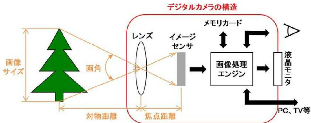
付録1-図1.3 デジタルカメラの仕組み
