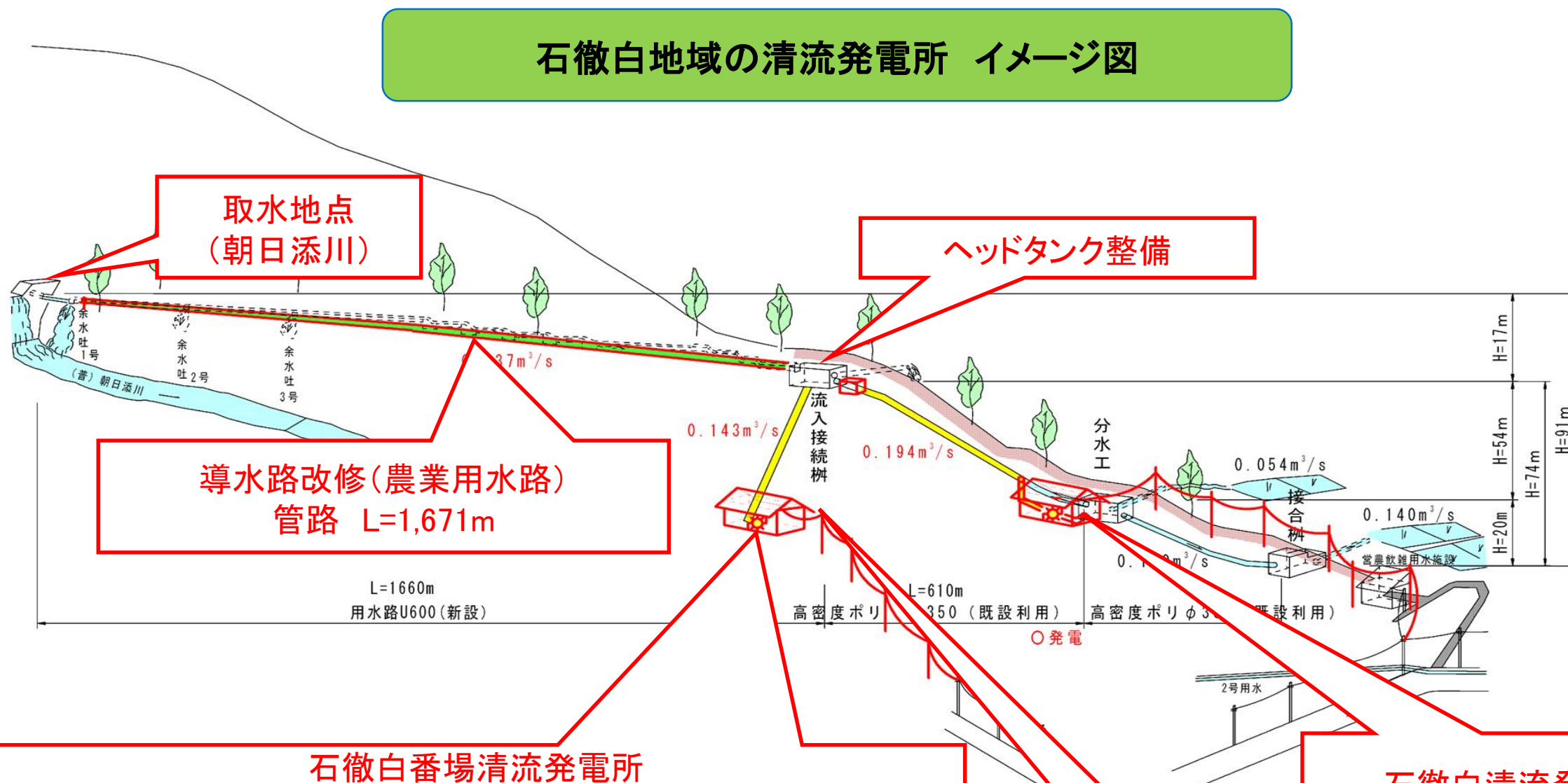
石徹白清流発電所 63kW(石徹白地区)
