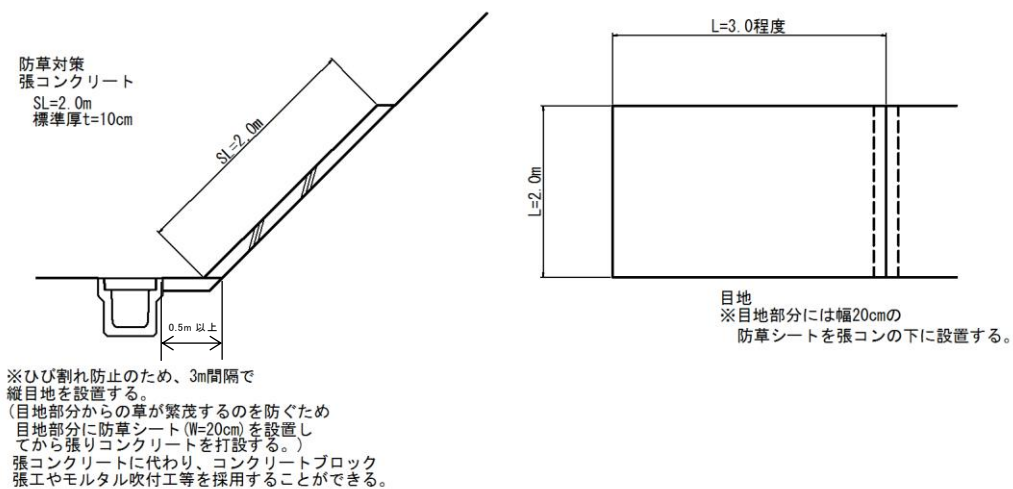
図 4.1.40 法面（法尻）（県仕様）
