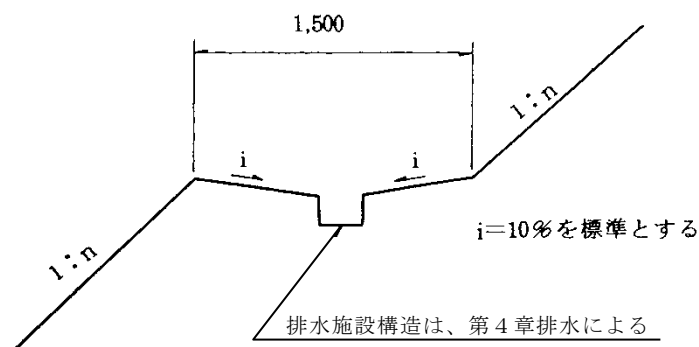
図 4.1.6 盛土の小段
