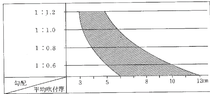
図 4.1.28 勾配と平均吹付圧の目安
