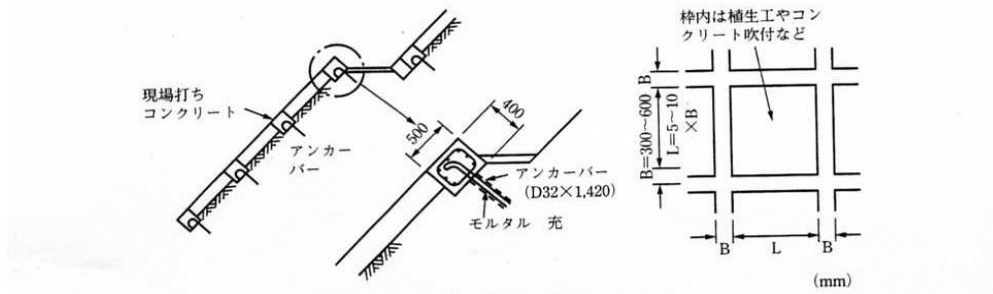
図 4.1.34 現場打ちコンクリート枠工の例（1）
