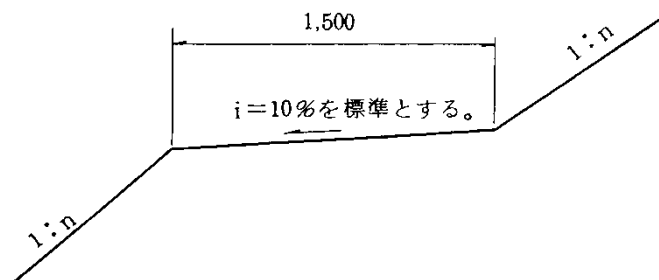
図 4.1.7 盛土の小段
