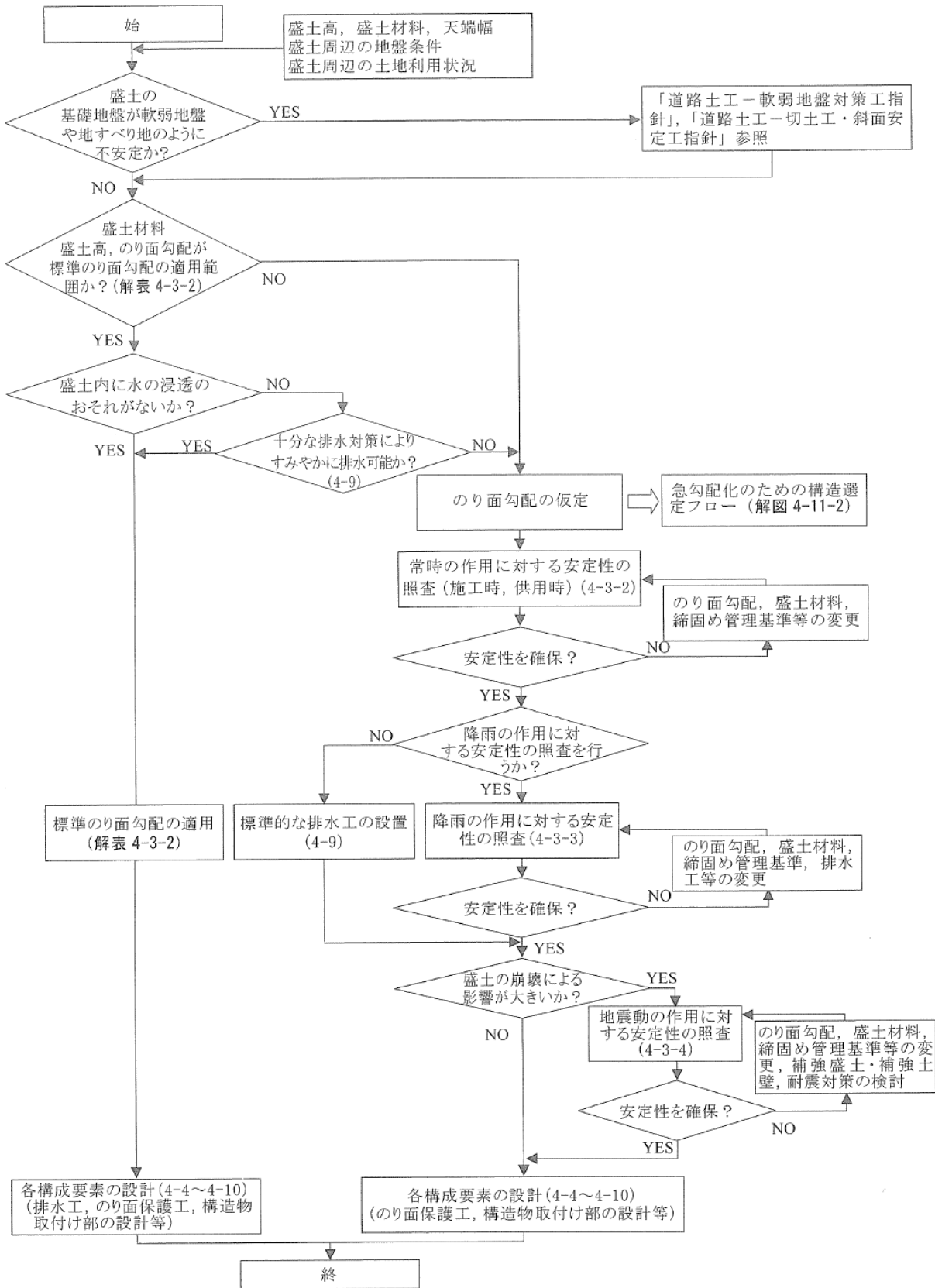
図 4.1.2 盛土の安定性照査のフローチャートの例 (土工、盛土 H22 p104)
