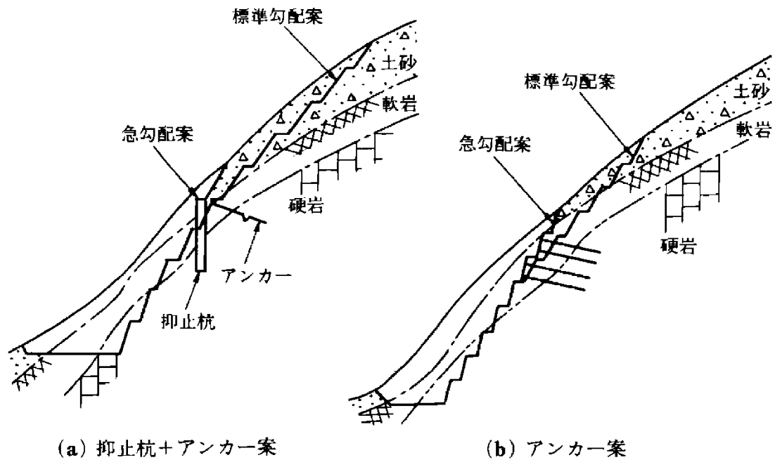
図 4.1.11 急傾斜地の切土
