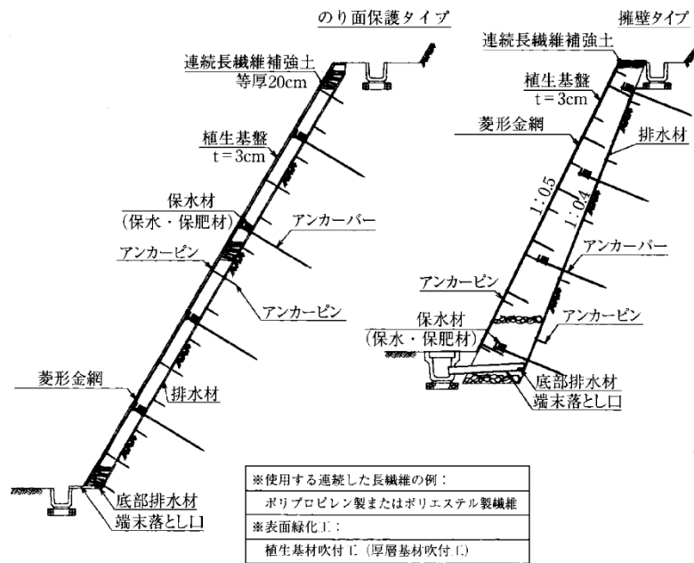
図 4.1.36 連続長繊維補強土工の例
