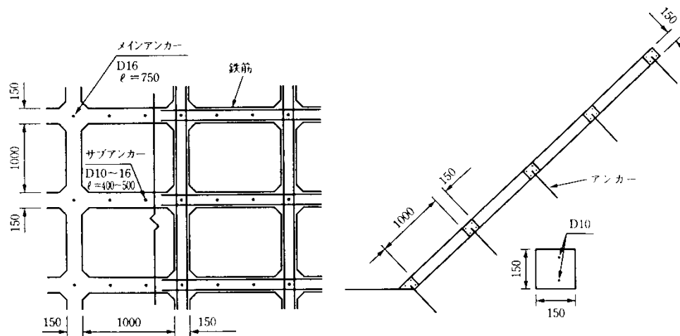
図 4.1.32 吹付枠工の例
