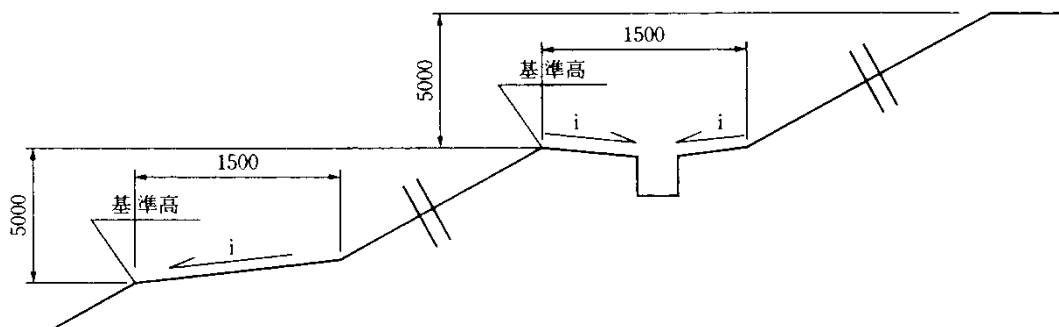
図 4.1.8 盛土高の基準位置
