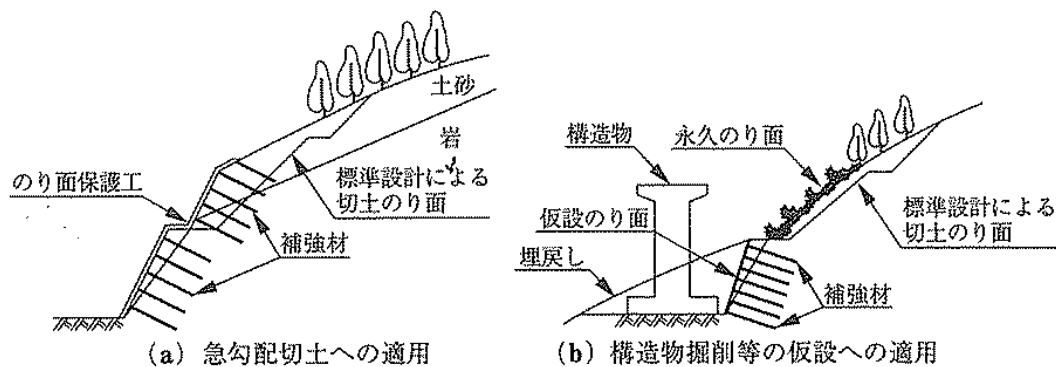
図 4.1.37 鉄筋挿入工の適用例
