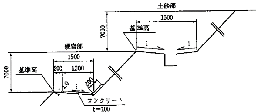
図 4.1.14 切土高の基準位置
