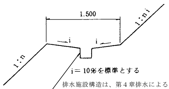
図 4.1.13 切土の小段 詳細図
