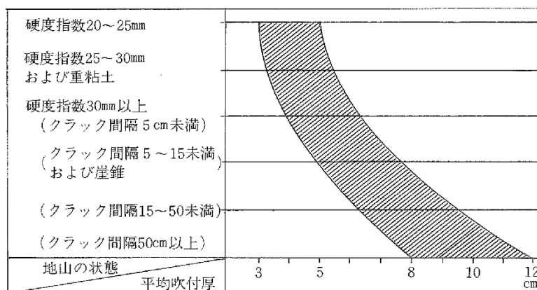
図 4.1.26 地山の状態と平均吹付厚の目安
