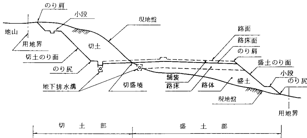
図 4.1.1 各部の名称
