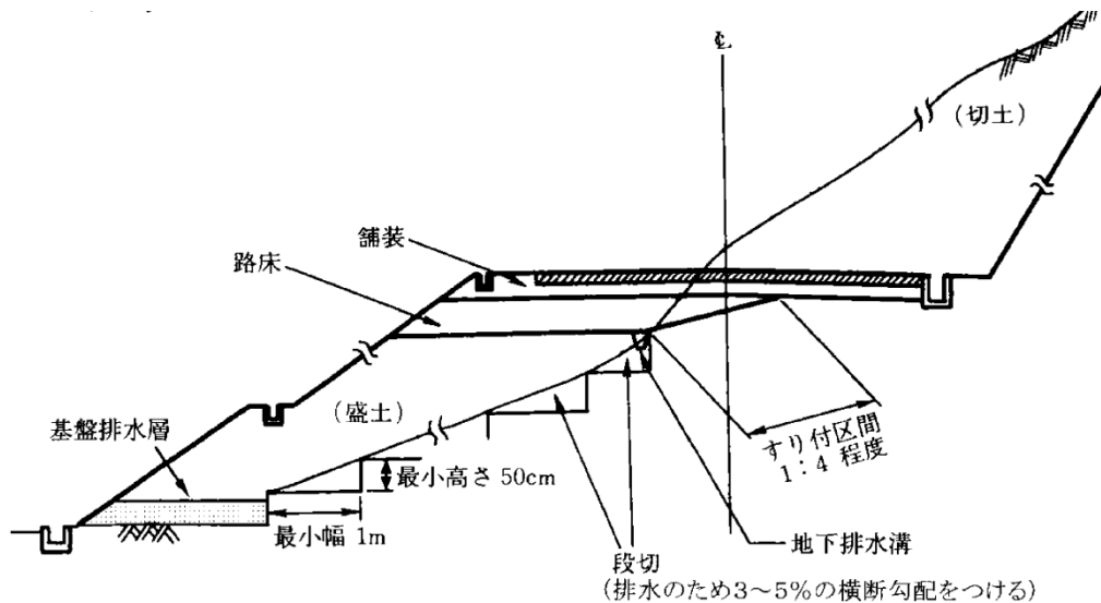
図 4.1.18 段切り、片切り、片盛りの摺付
