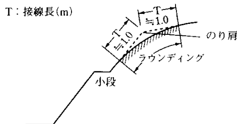
図 4.1.15 ラウンディングの範囲
