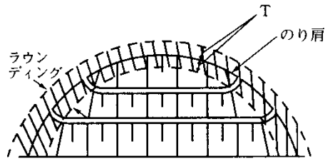
図 4.1.16 縦断方向のラウンディング
