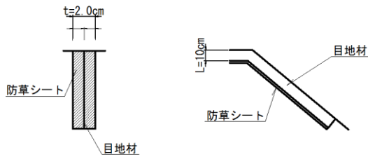
目地部詳細図
