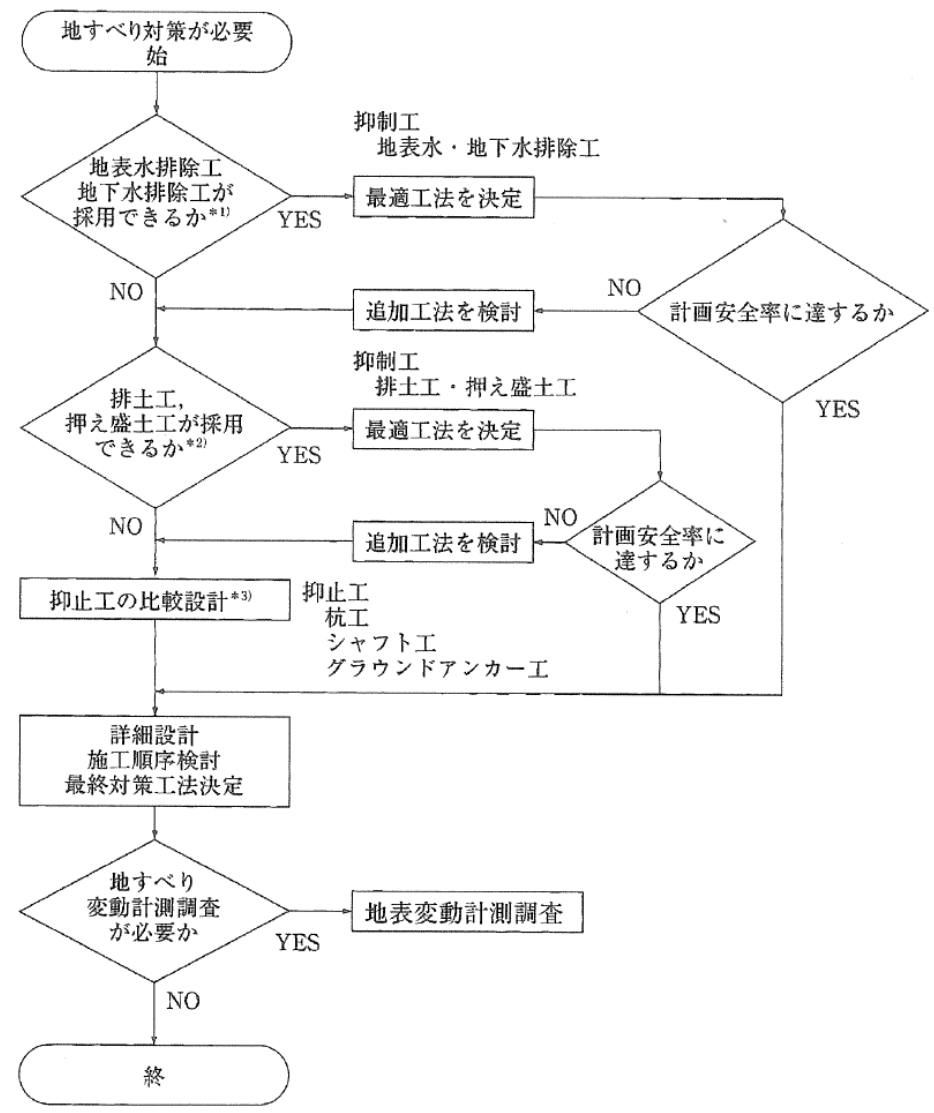
図 4.1.43 地すべり対策工検討フローチャート (土工、斜面 H21 p405)
