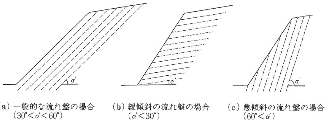
図 4.1.10 流れ盤における割れ目とのり面の関係
