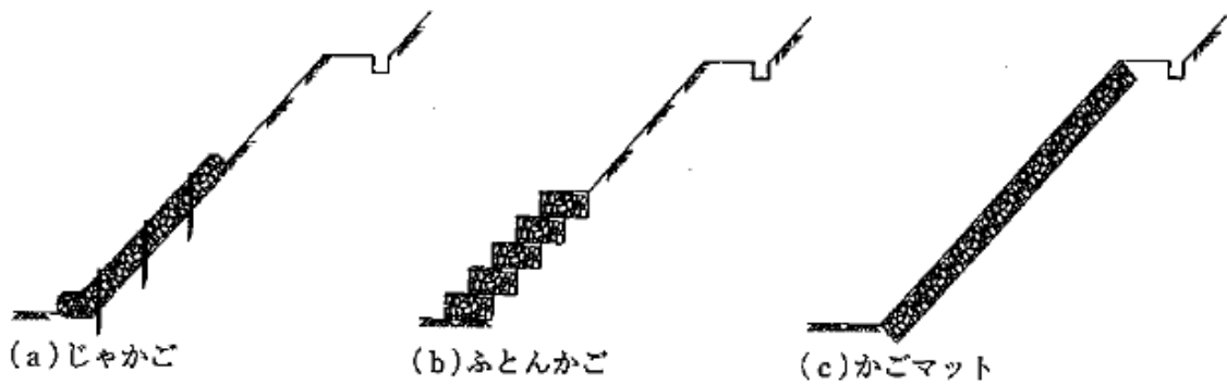
図 4.1.38 かご工の一般形状例
