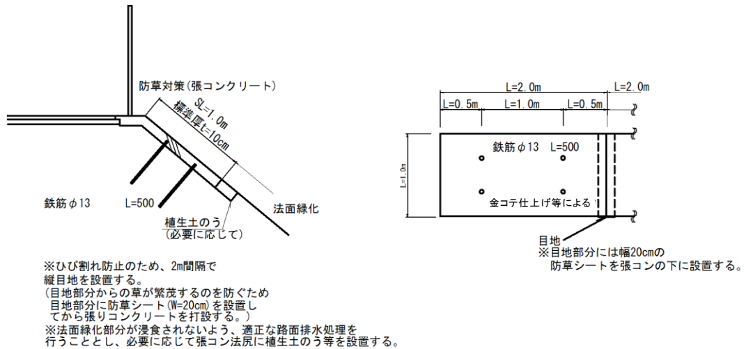
目地部詳細図
