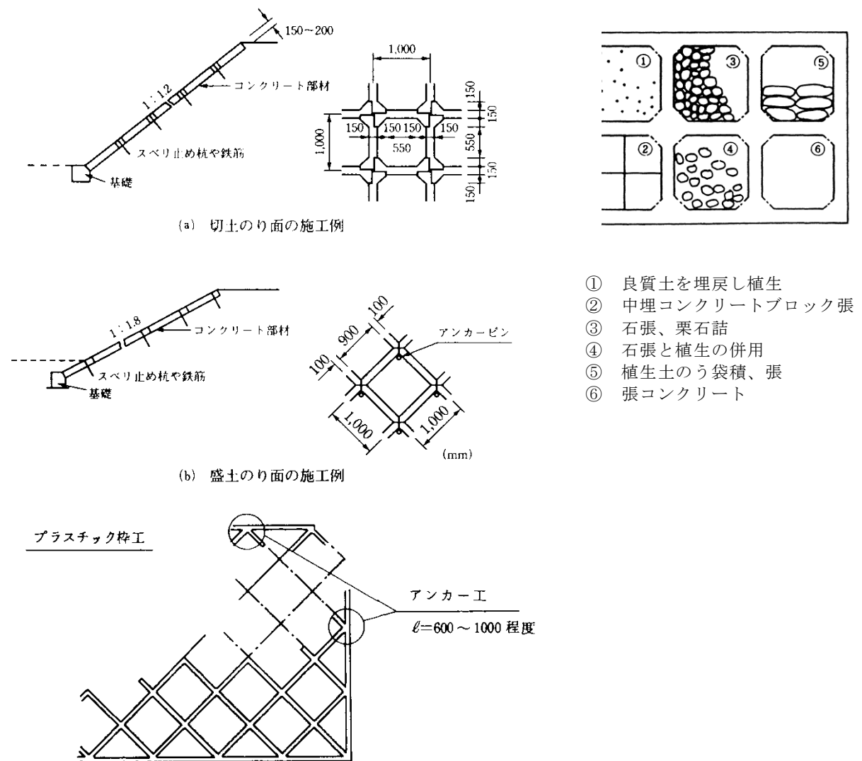
図 4.1.31 コンクリートブロック枠工の例
