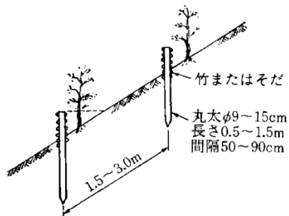
図 4.1.29 柵の一部を表面に出す場合
