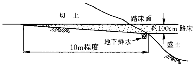
図 4.1.19 切土部路床に置換え盛土のない場合
