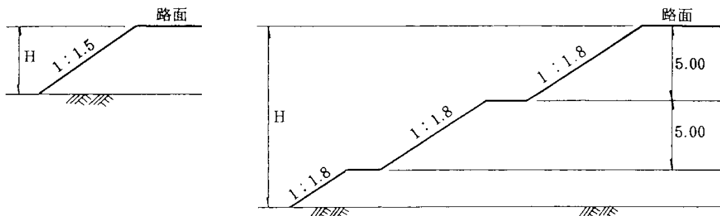
図 4.1.3(a) 盛土のり面勾配標準図 (本線)
