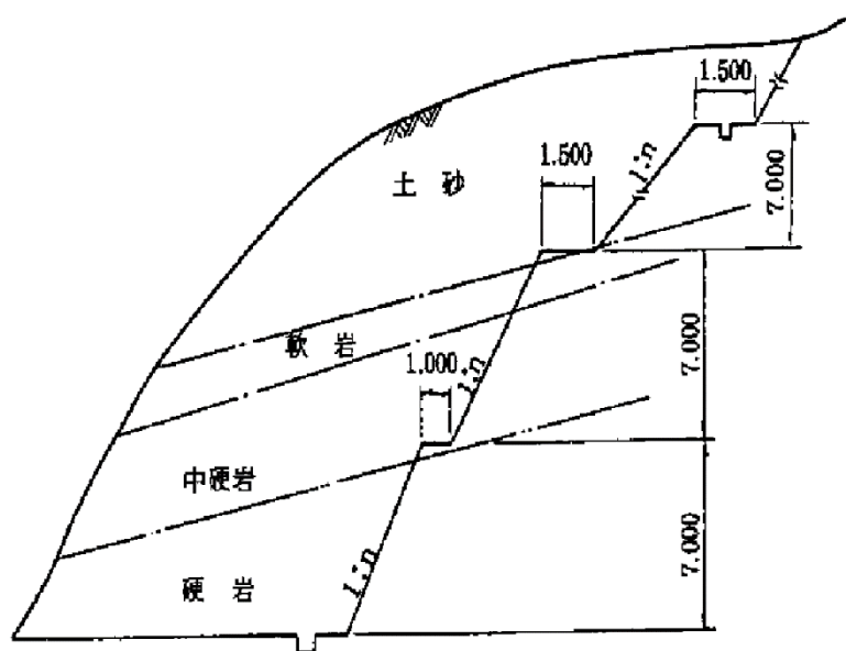
図 4.1.12 切土の小段
