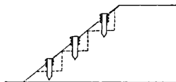
図 4.1.30 段切による柵工の設置
