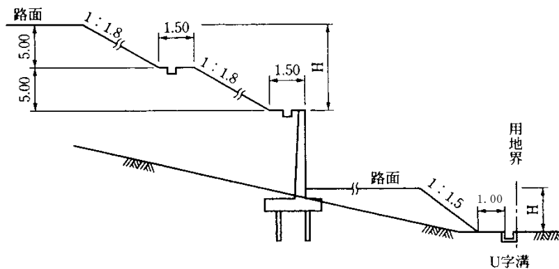
図 4.1.5 盛土の小段
