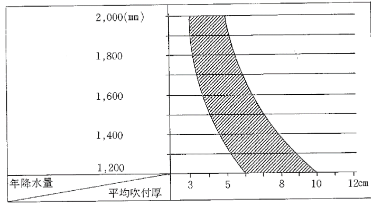
図 4.1.27 年降水量と平均吹付圧の目安
