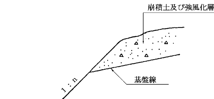
図 4.1.9 崩積土、強風化斜面切土の場合
