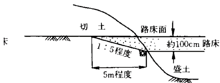
図 4.1.21 原地盤が岩で擦り付け区間を長くすることが不経済となる場合
