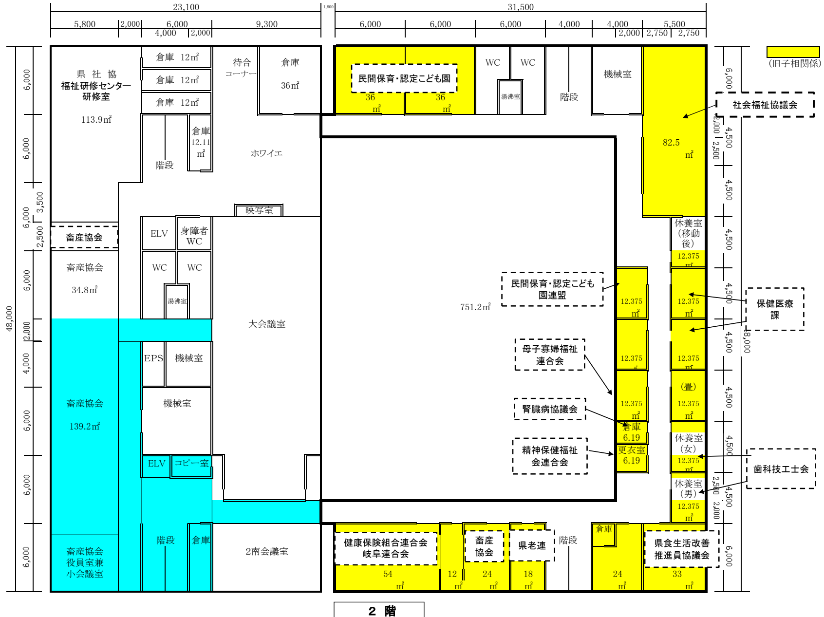
福祉・農業会館 平面図
