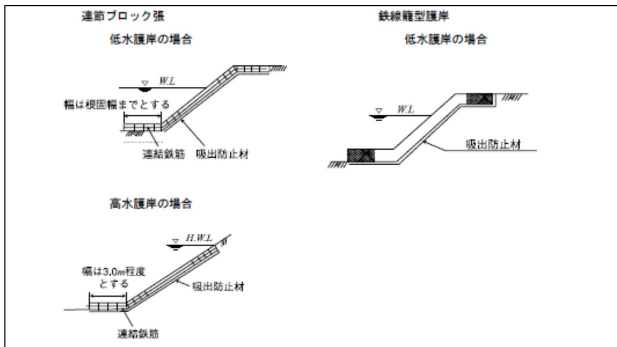
図 1-7 吸出し防止材の布設位置
