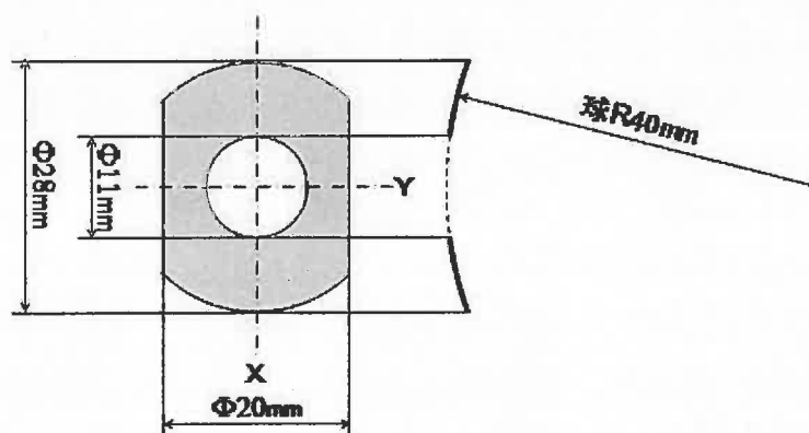
図 3 音場の計測値と数値計算値との比較により推定した集束超音波トランスデューサの寸法定数
